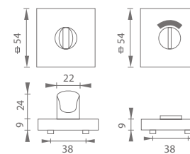
HR WC S UKAZOVATELOM
