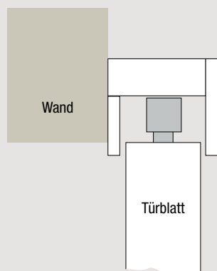
Montage auf der Wand ohne Zarge
