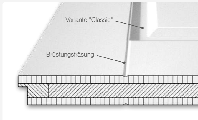
Querschnitt: 3-schichtiger Türblattaufbau
