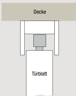
Montage unter der Decke
